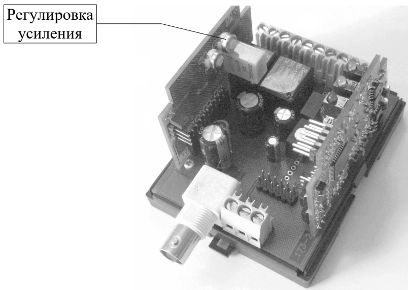
Рисунок 15. Изделие со снятой крышкой
