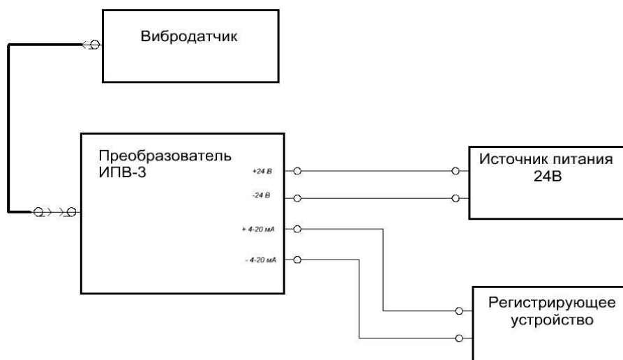
Рисунок 4. Схема подключения
