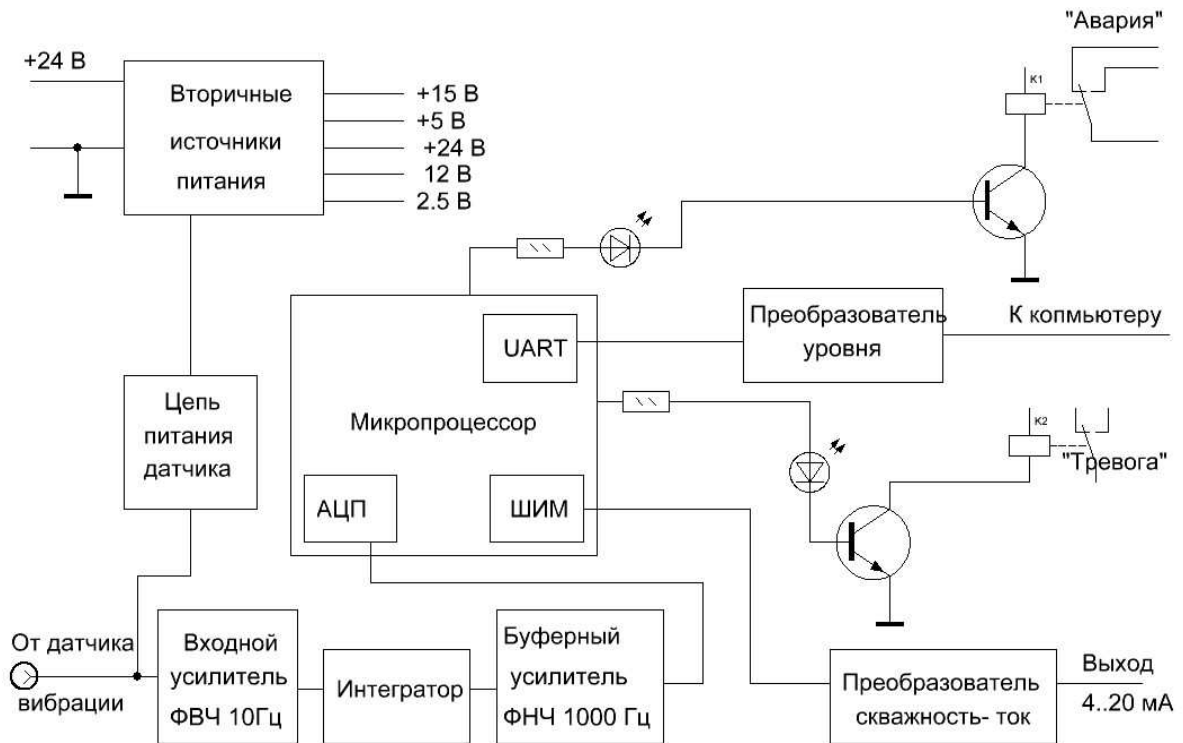
Рисунок 3. Структурная схема устройства
